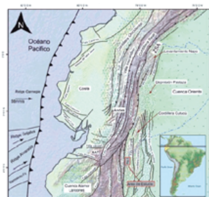
Figura 4. Esquema morfo tectónico del Ecuador. (Torres, et al., 2021)
