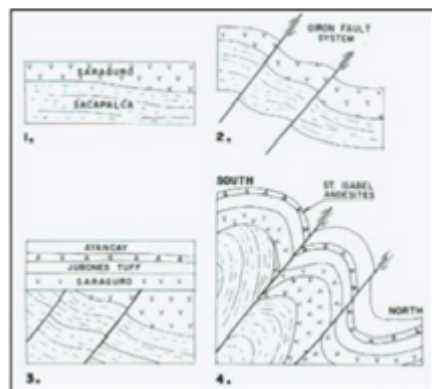
Figura 5. Desarrollo a lo largo de la historia del Sistema de Fallas Girón, las imágenes muestran el siguiente proceso: 1. Antes de 23 Ma. 2. después de 23 Ma. 3. después de 14 Ma. 4. Hoy en día (CODIGEM, 1997 cómo se citó en Ávila, 2020)
