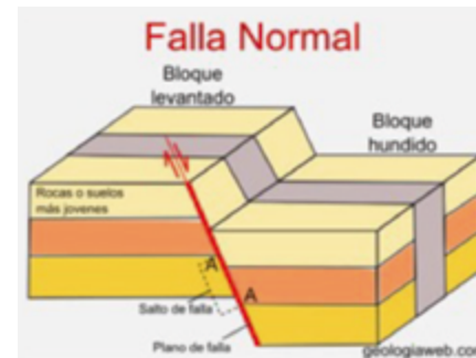
Figura 2. Modelo de comportamiento de falla Normal (geologiaweb, s.f)
